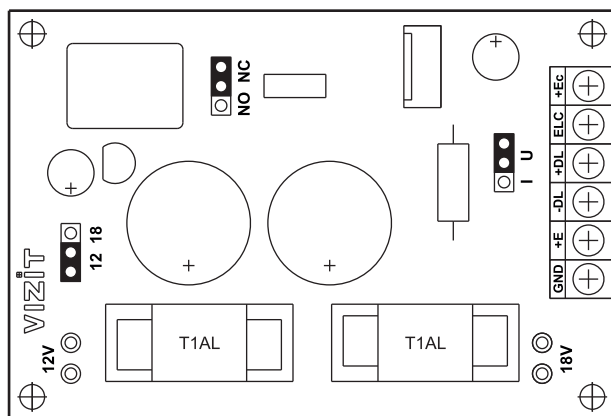
Рисунок 1 - Расположение элементов на плате блока питания ВПД18/12-3-1
